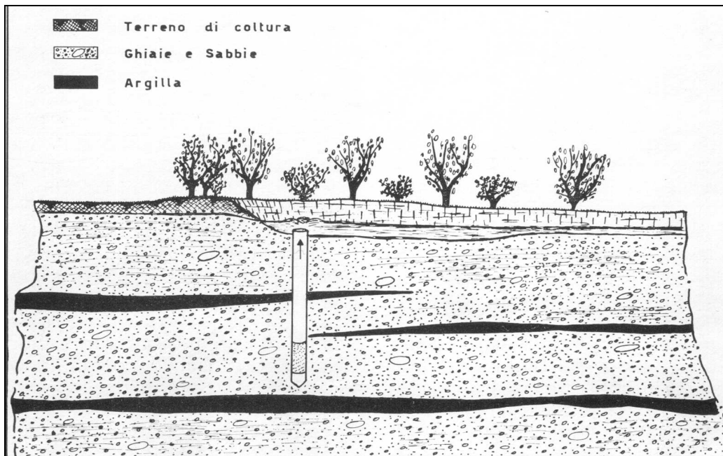
Figura 3.7 - sezione di un fontanile
