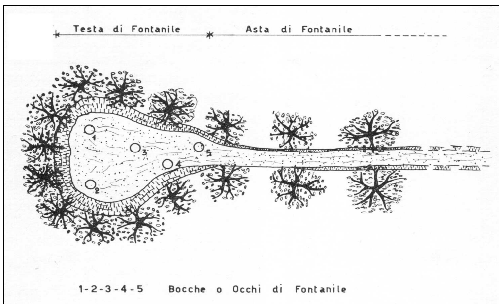
Figura 3.6 - pianta di un fontanile
